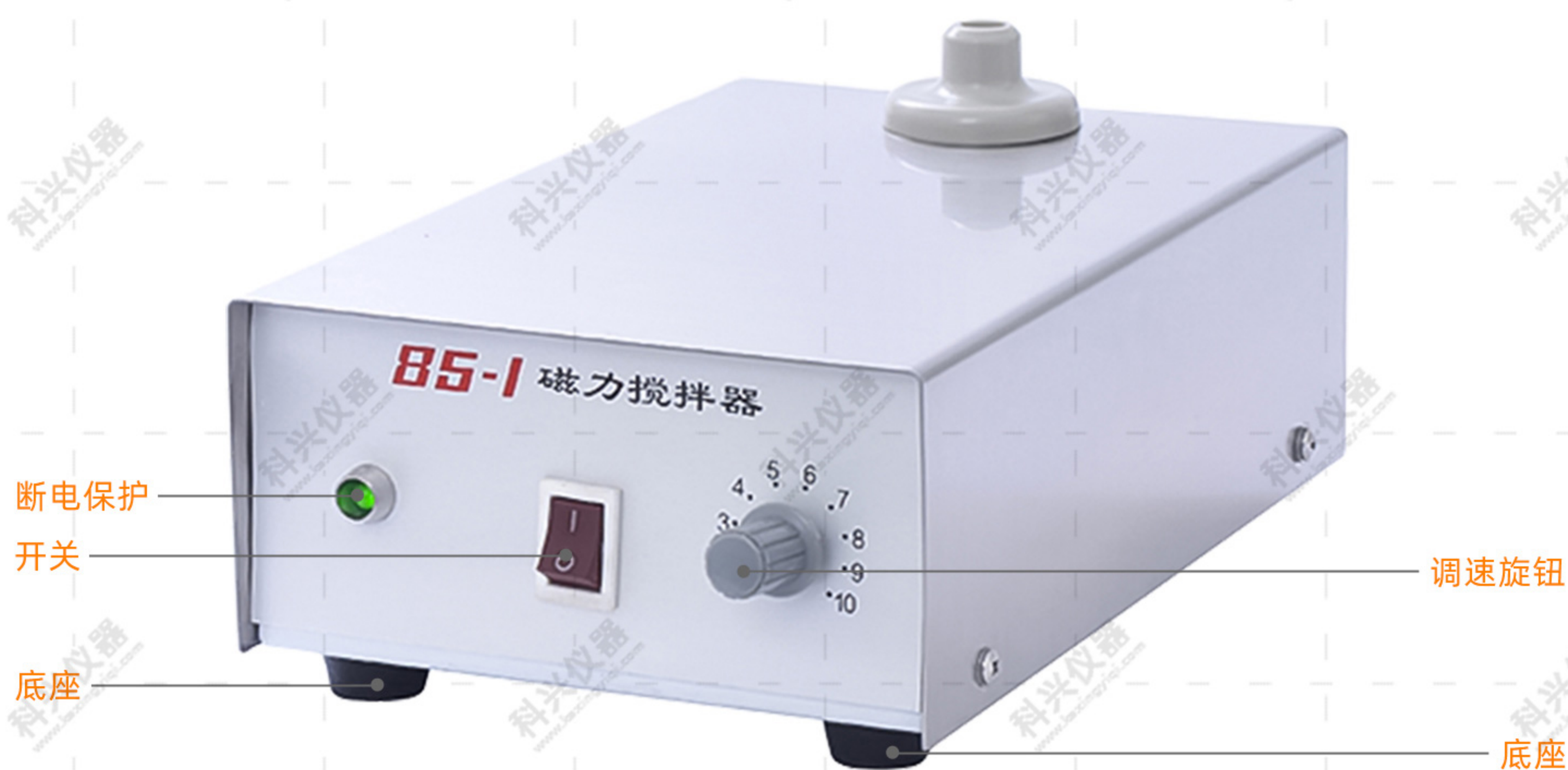
85-1型磁力搅拌器
